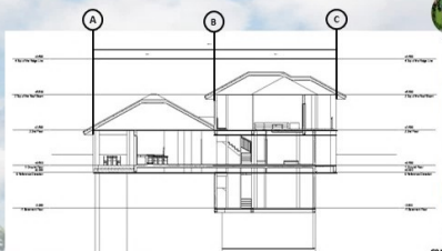
LONGITUDINAL SECTION THRU X1-X2 SCALE: 1:500 MTS
