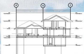
LONGITUDINAL SECTION THRU Y1-Y2 SCALE: 1:500 MTS
