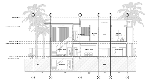
S-01 LONGITUDINAL SECTION 1:150
