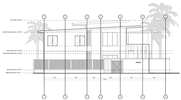
LEFT ELEVATION 1:150
